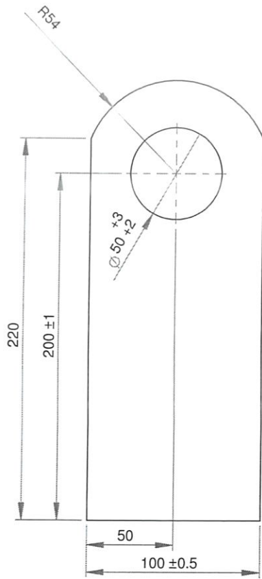
SCALE 1 : 3
