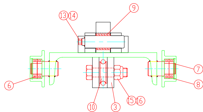
SECTION A-A SCALE 1 : 2
